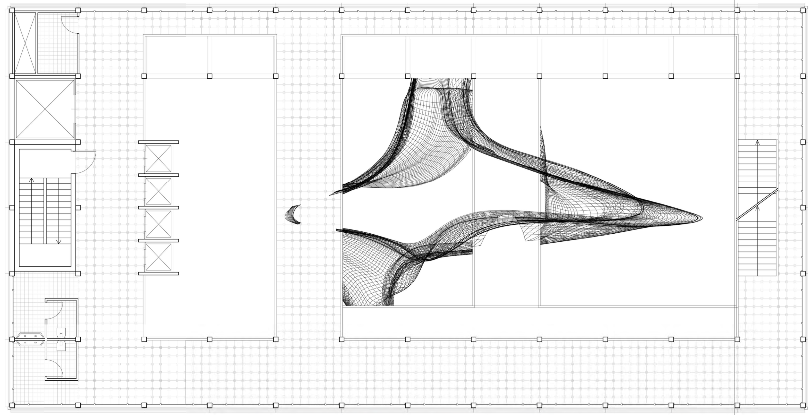
PIANTA LIVELLO 11 SCALA 1:100
