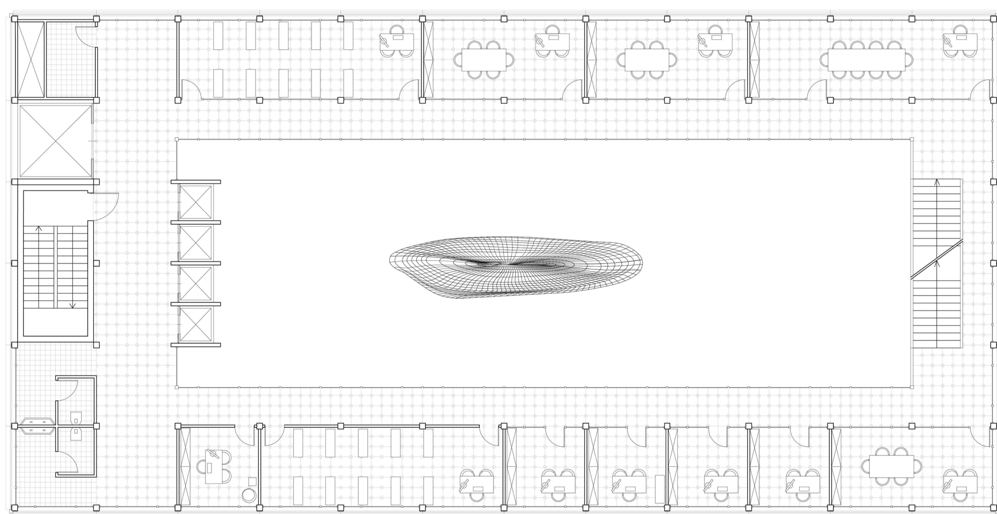
PIANTA LIVELLO 3
