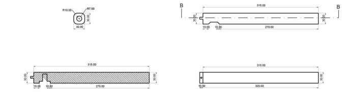
SEZIONE B_B
