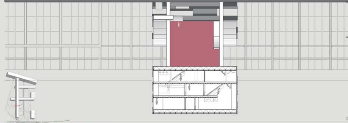
SEZIONE alloggi, scala 1:200
