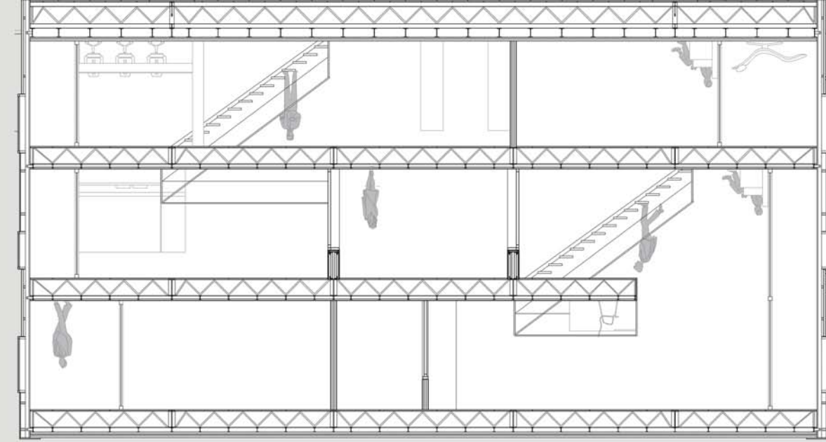
SEZIONE alloggi, scala 1:200
