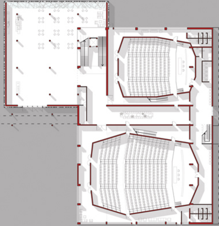
sezione orizzontale +2m scala 1:200
