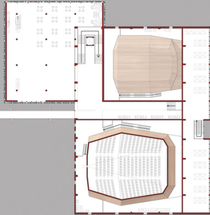
sezione orizzontale +8m scala 1:200
