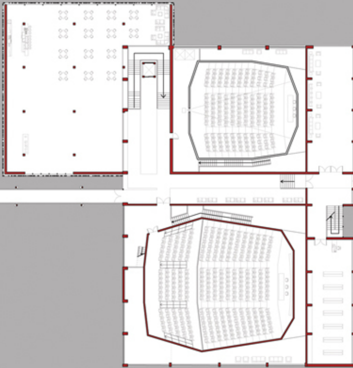
sezione orizzontale +5m scala 1:200
