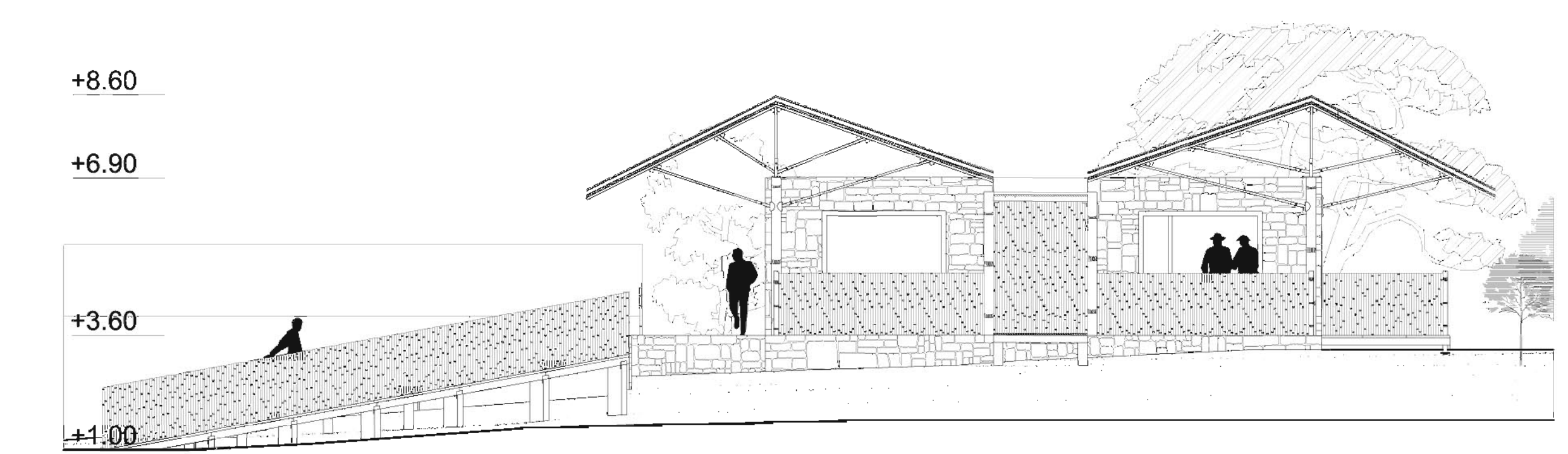
prospetto EST scala 1:100
