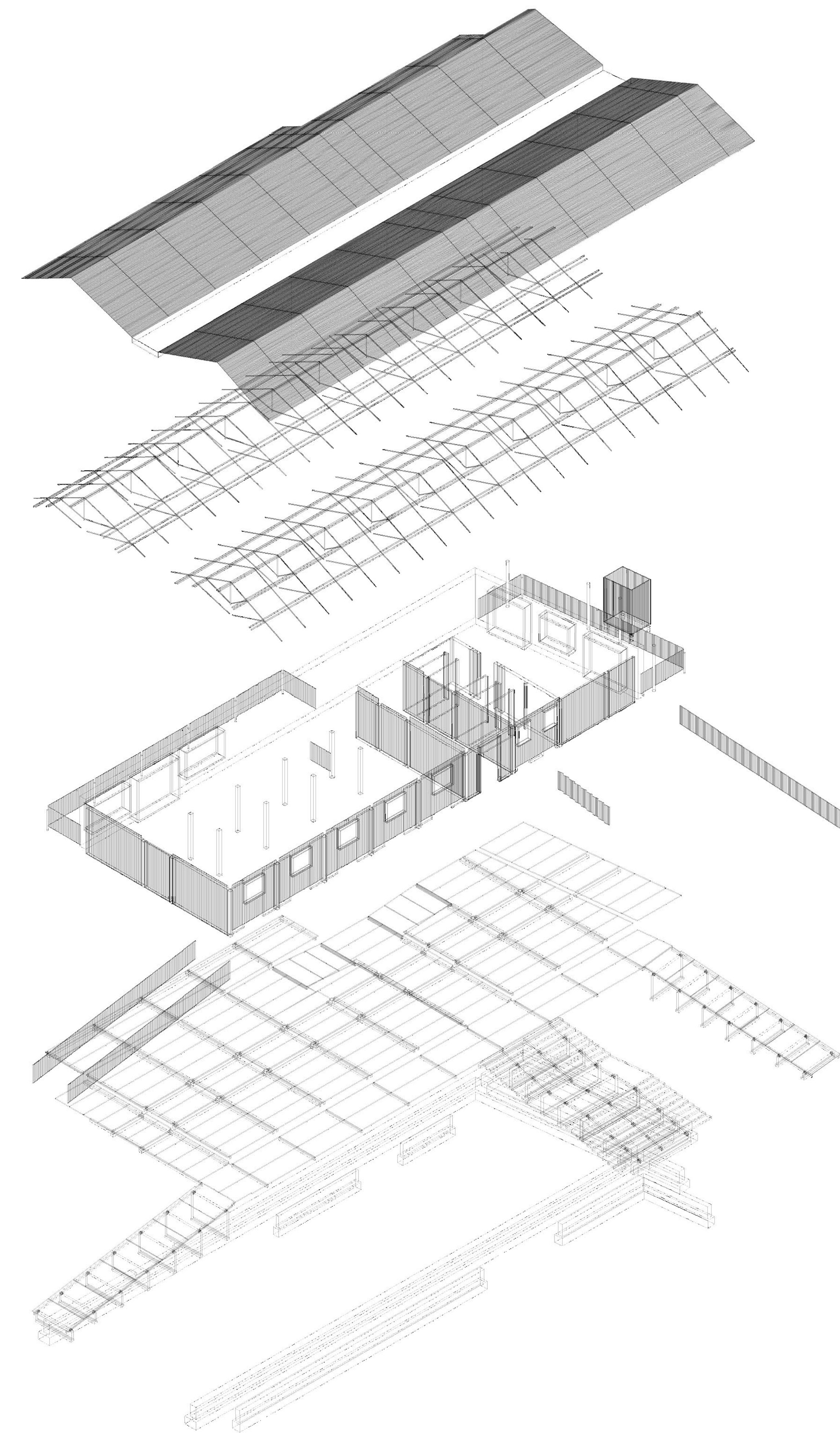
esploso assometrico
