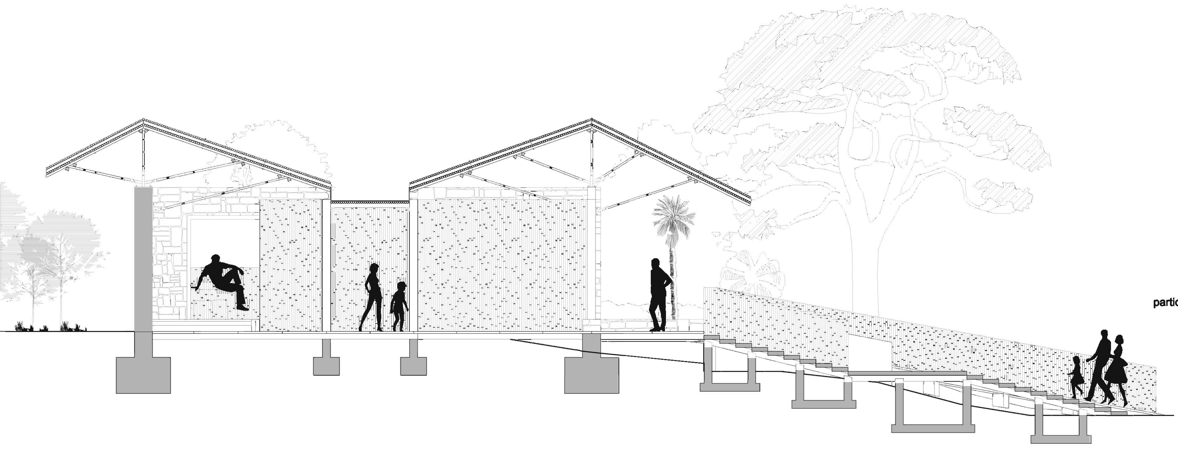
sezione BB' scala 1:100
