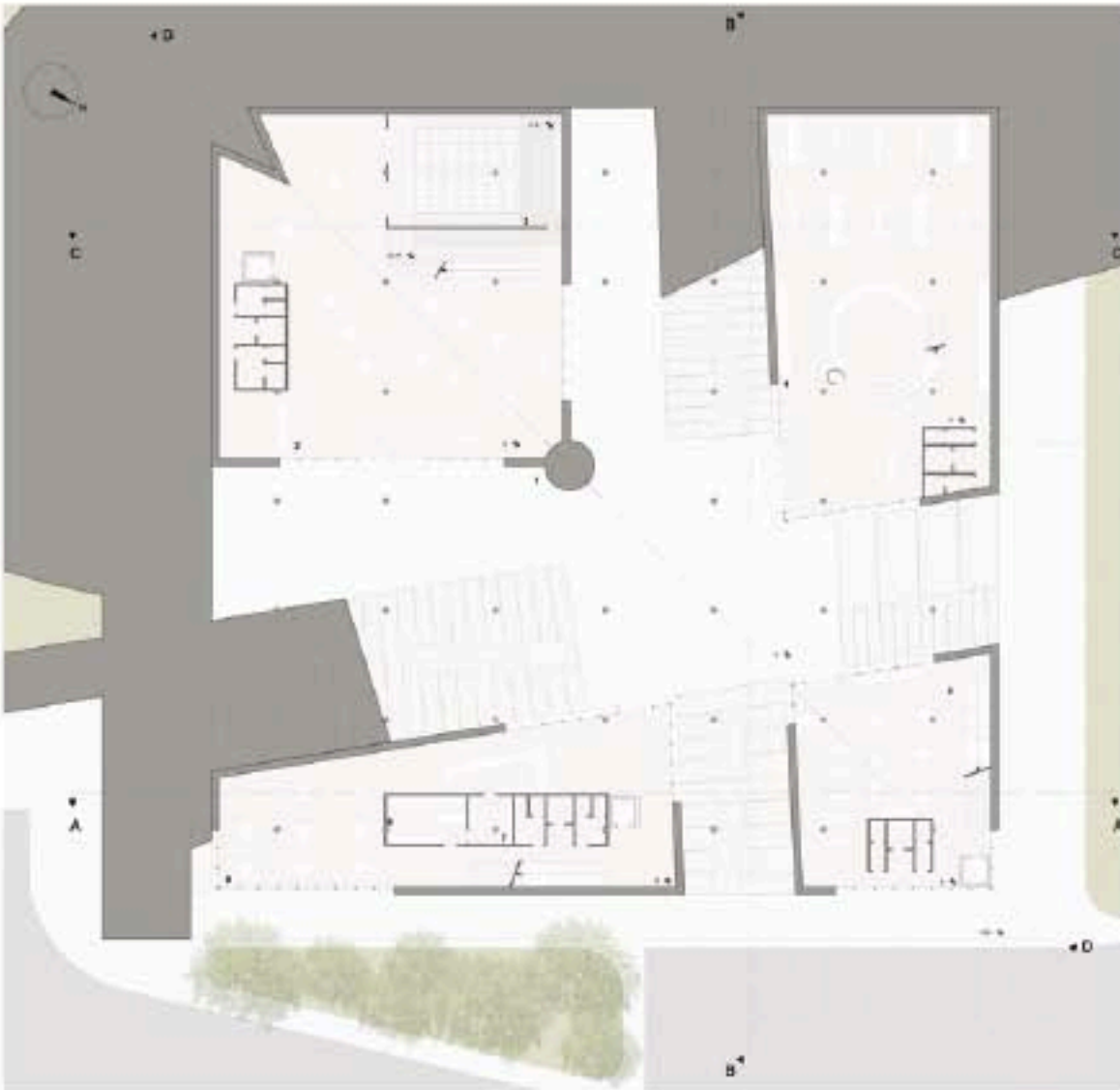
Pianta Secco 1°, 1/200
