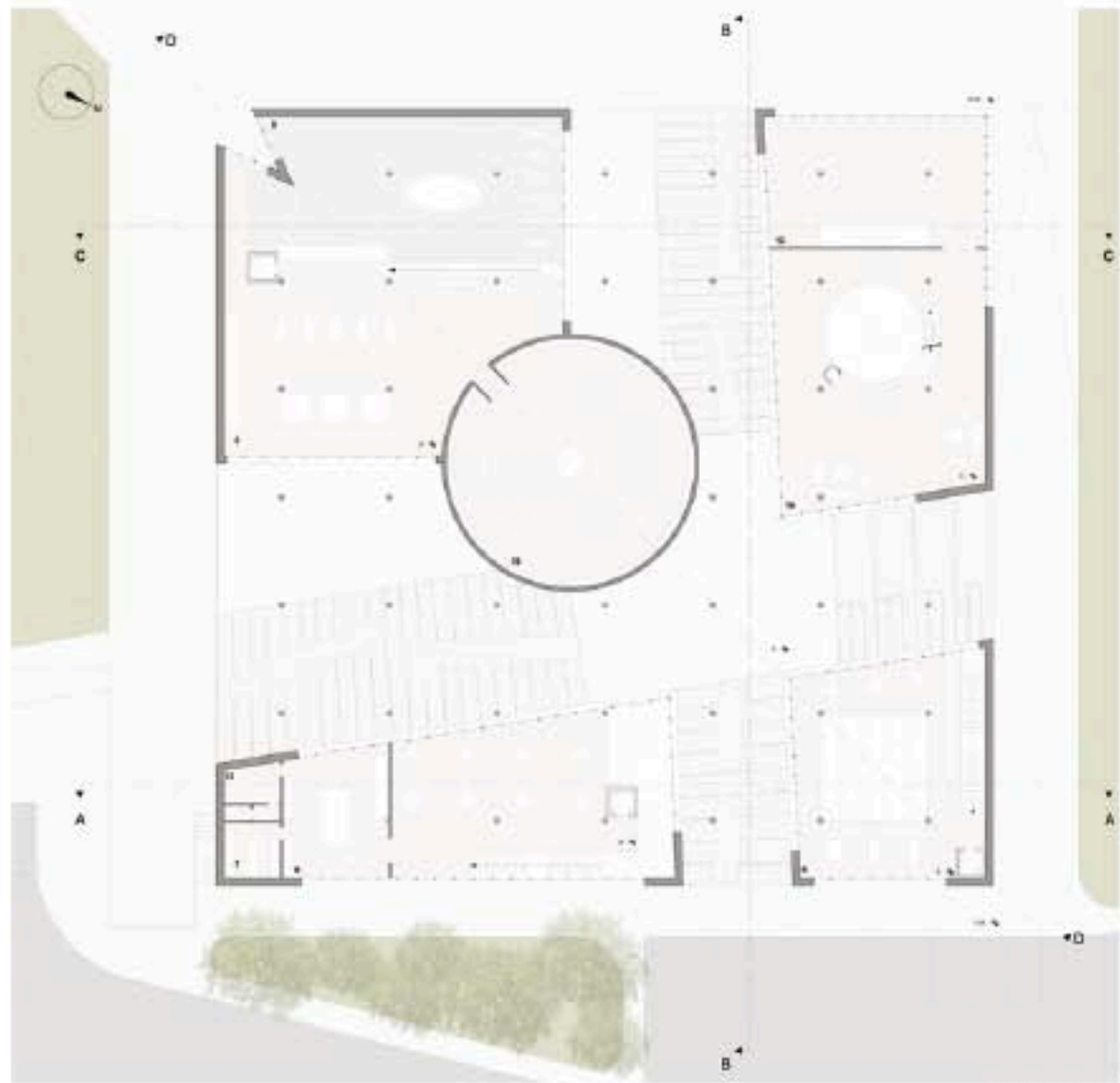
Pianta livello 2°_1:200
