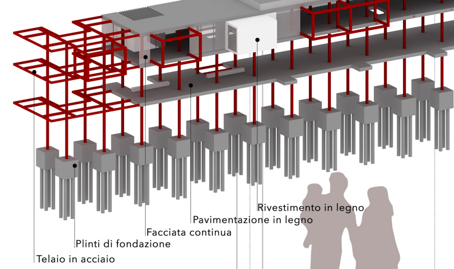
Schema strutturale
