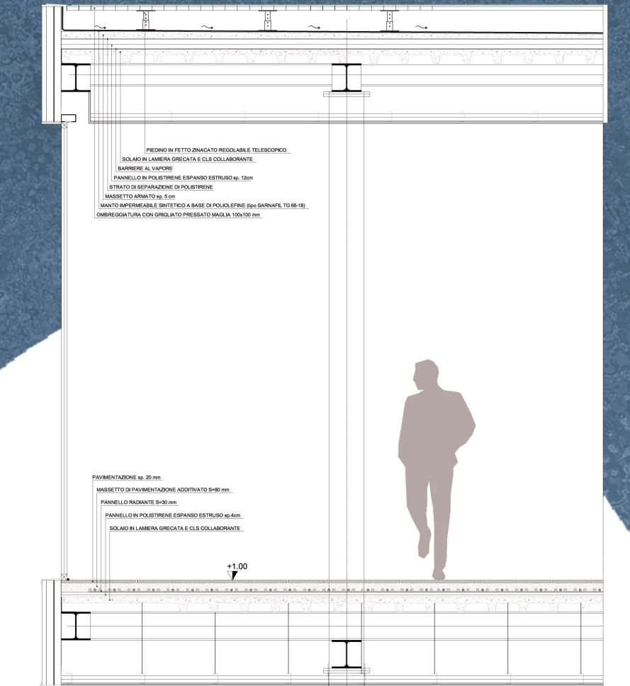
Sezione tipologica B-B scala 1:20
