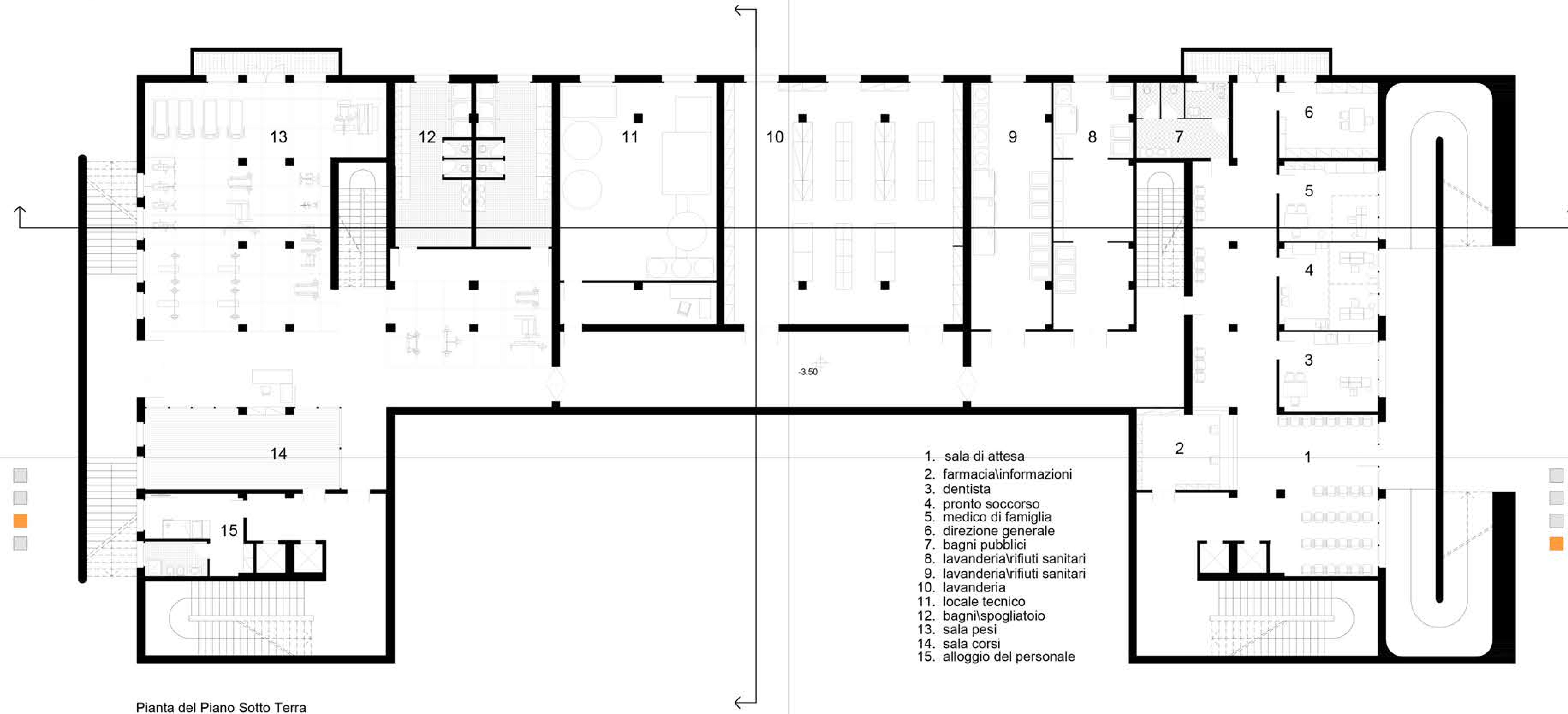
Pianta del Piano Sotto Terra
