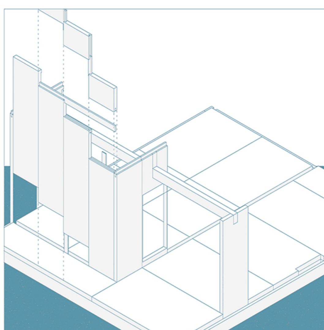
MONTAGGIO PAVIMENTO
