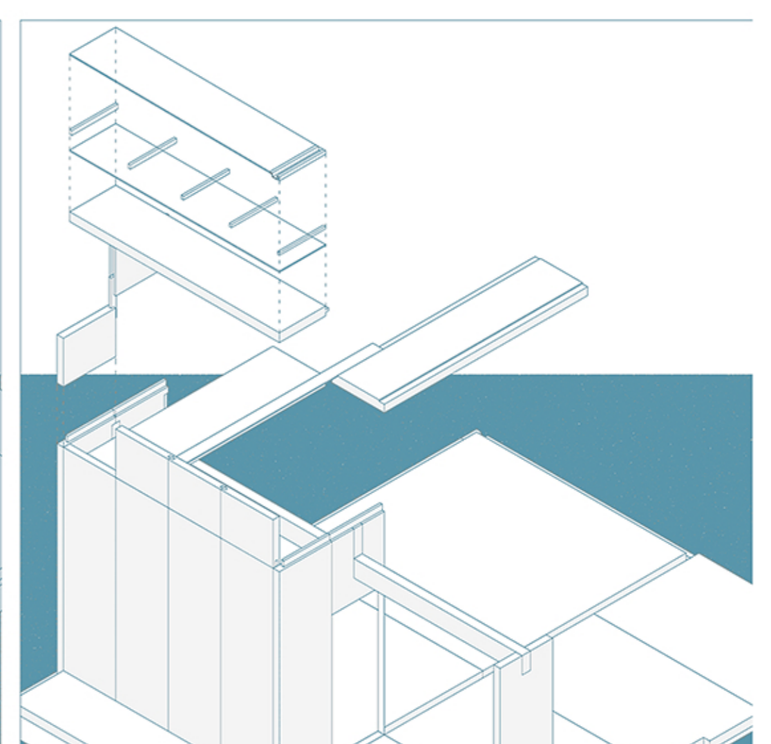
MONTAGGIO PARETI
