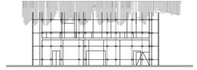
PROSPETTO SUD
