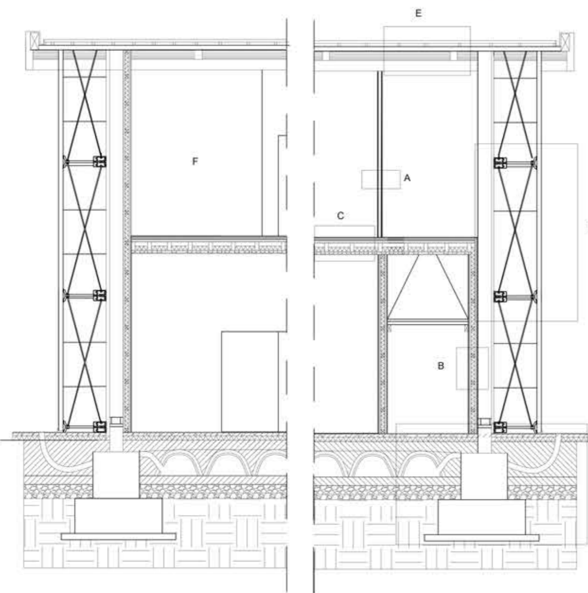
A PARTIZIONE DIVISORIA INTERNA A SECCO Fermacell - lastre in gessofibra, 12,5 mm Pavatex PAVAFLEX 60 mm - pannello cobente flessibile in fibra di legno, interposto a profili metallici 75 mm Fermacell - lastre in gessofibra, 12,5 mm
