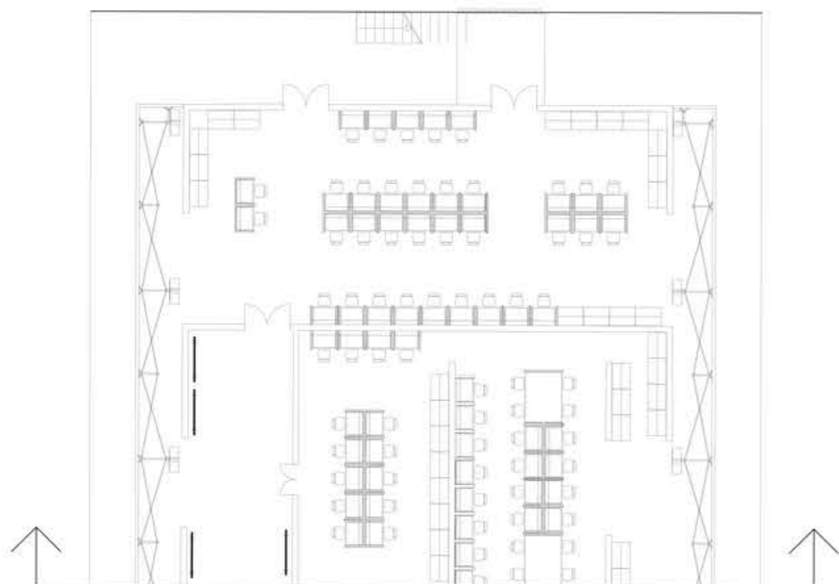
STRALCIO DI PIANTA PIANO TERRA 1:50
