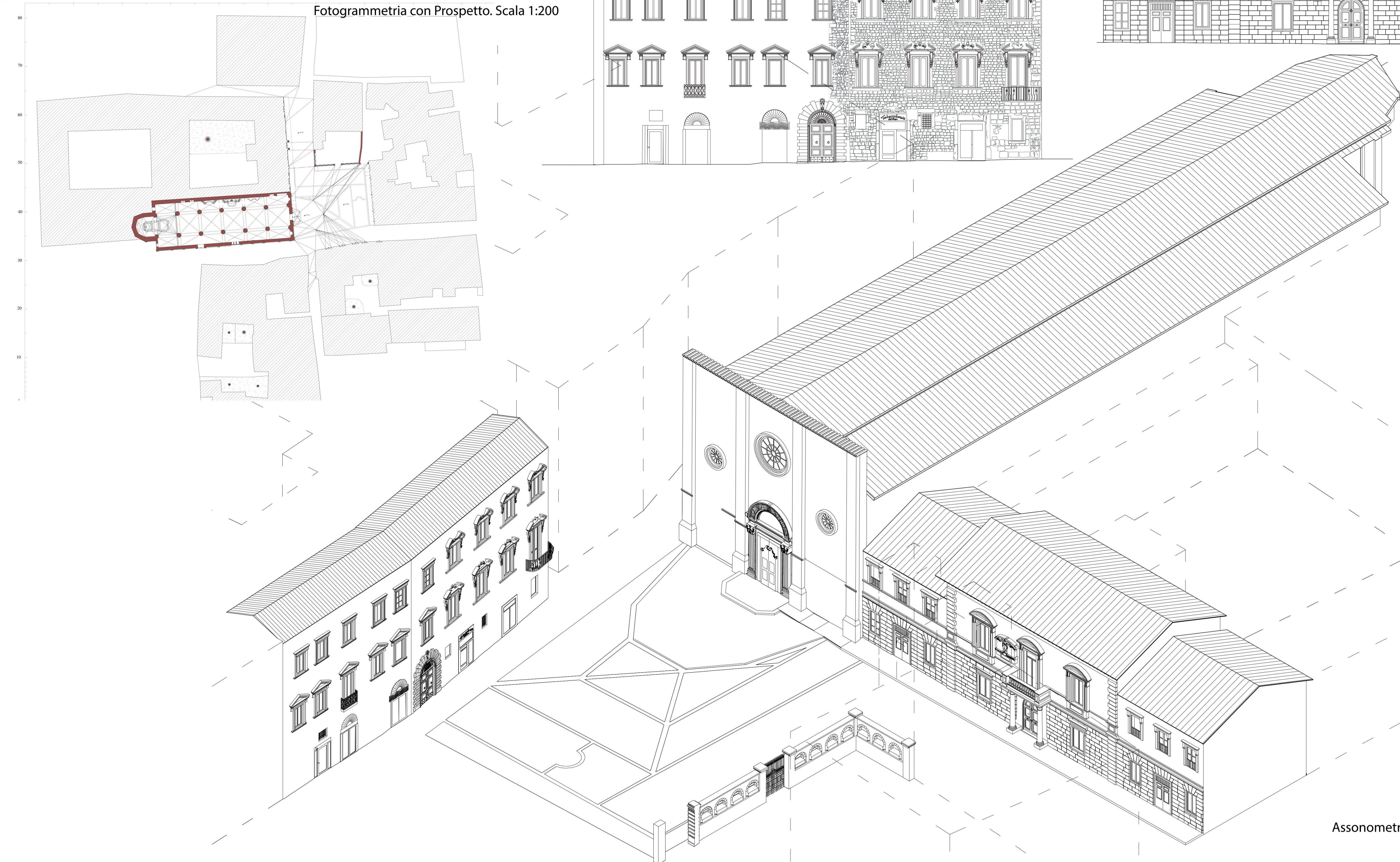
Fotogrammetria con Prospetto. Scala 1:200
