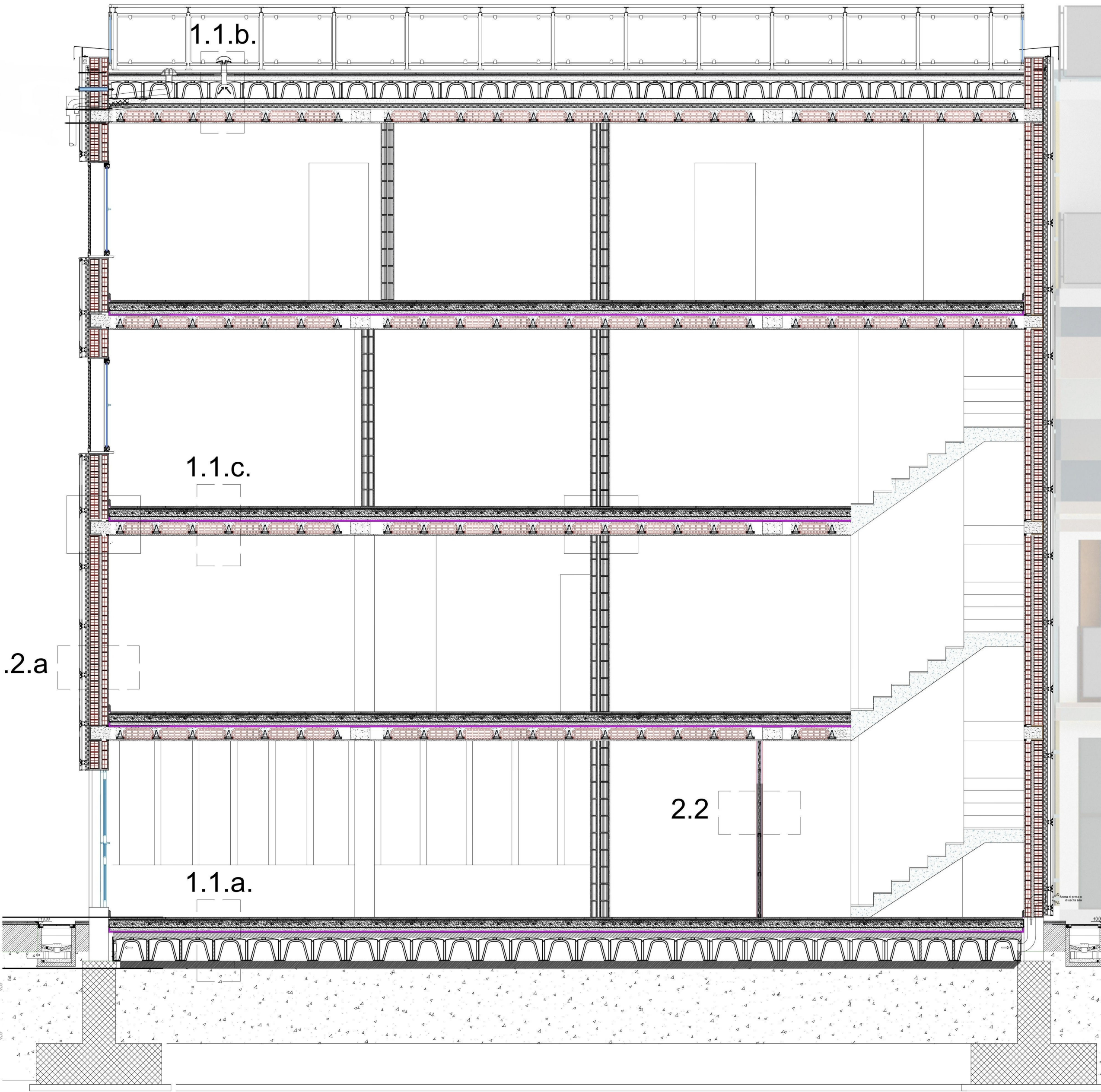
Sezione Stratigrafica. Scala 1:50
