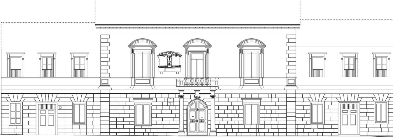
Fotogrammetria con Prospetto. Scala 1:200
